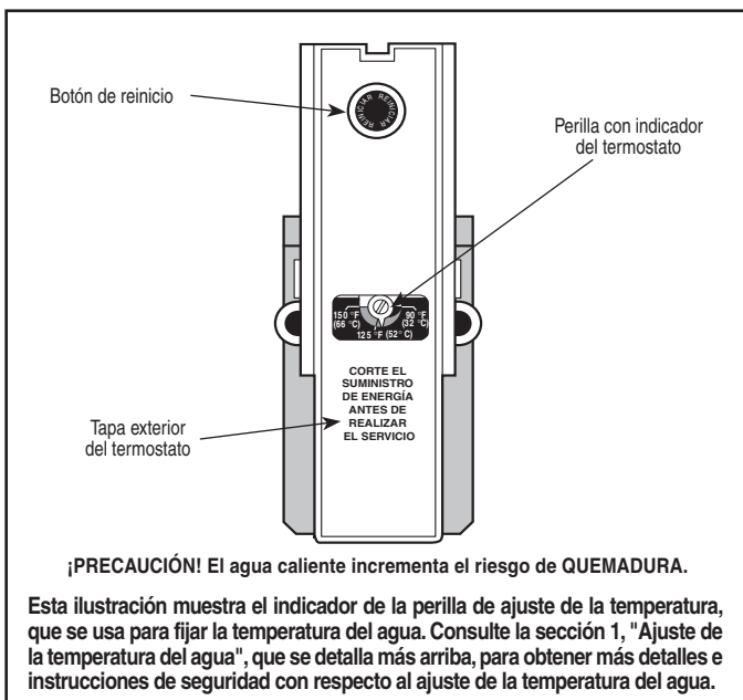
Figura 4: Cubierta del termostato y de protección
