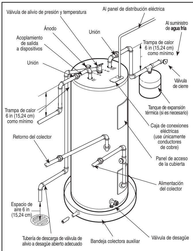
Figura 2: Instalación típica para los modelos de conexión lateral
