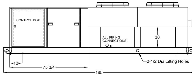
FAN CONFIGURATION "D"
